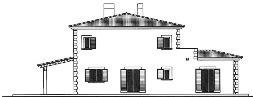
ALZADO LATERAL IZQUIERDO
